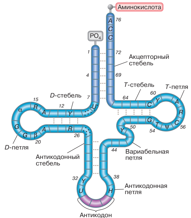
Рис. 2. Обобщенная вторичная структура молекул транспортных РНК (клеверный лист). Указаны основные фрагменты структуры: антикодон, ограниченный модифицированными нуклеотидами, выделяющими триплетную рамку; неспецифический участок АСС, связывающий аминокислоту; четыре двухспиральных участка (стебля) и три неспаренные петли
